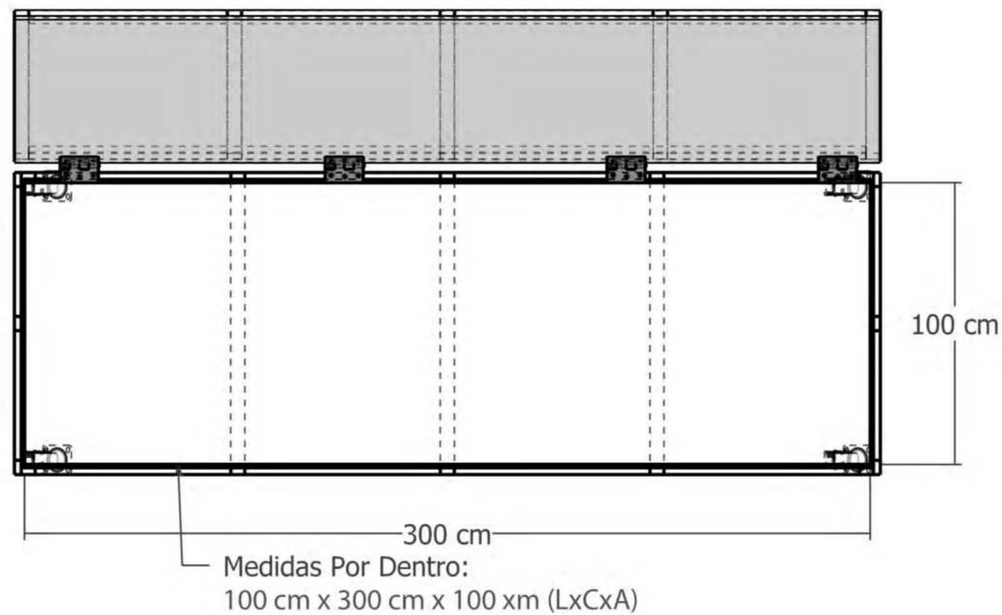
Case - Planta
