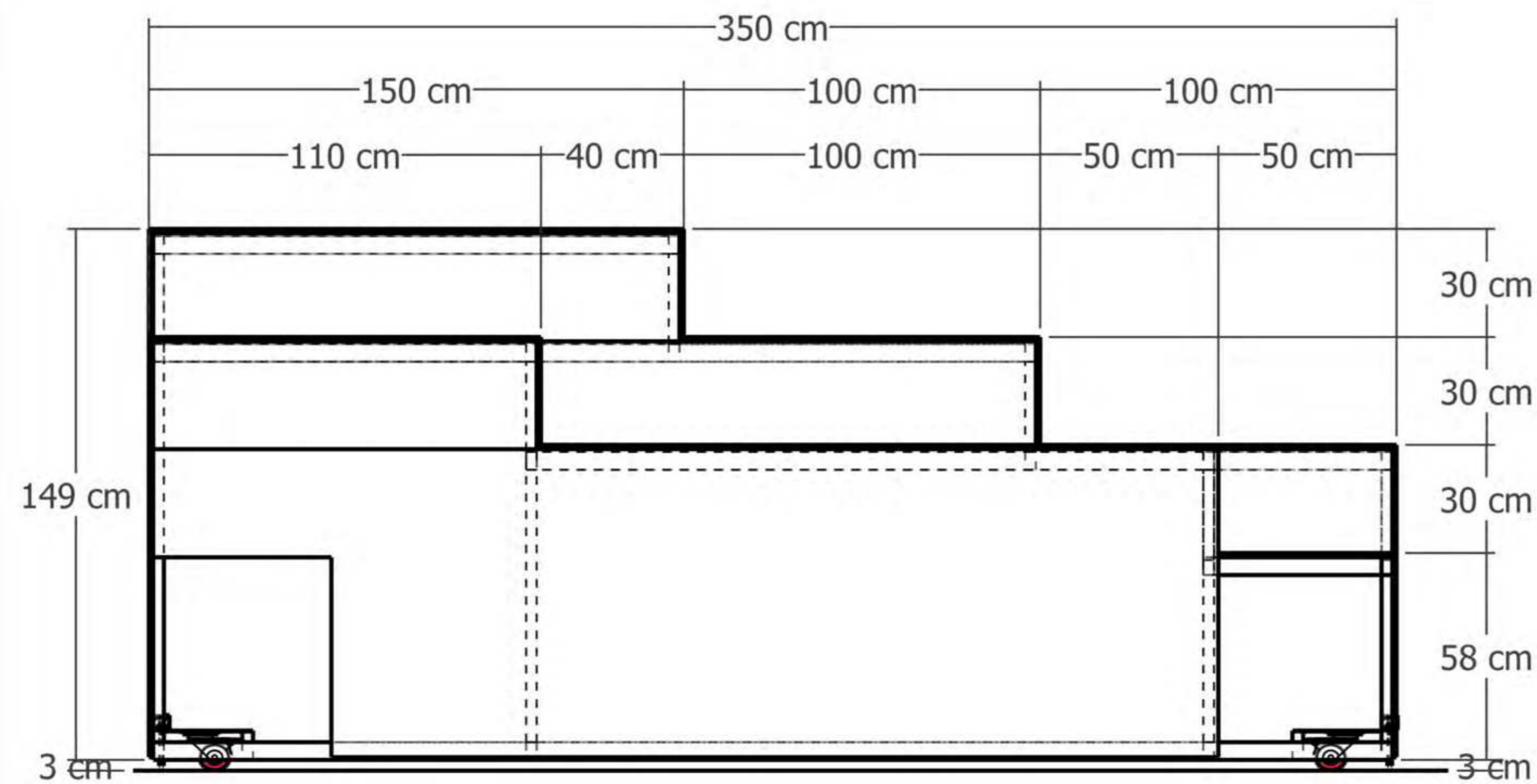
Peça B - Vista Frontal
