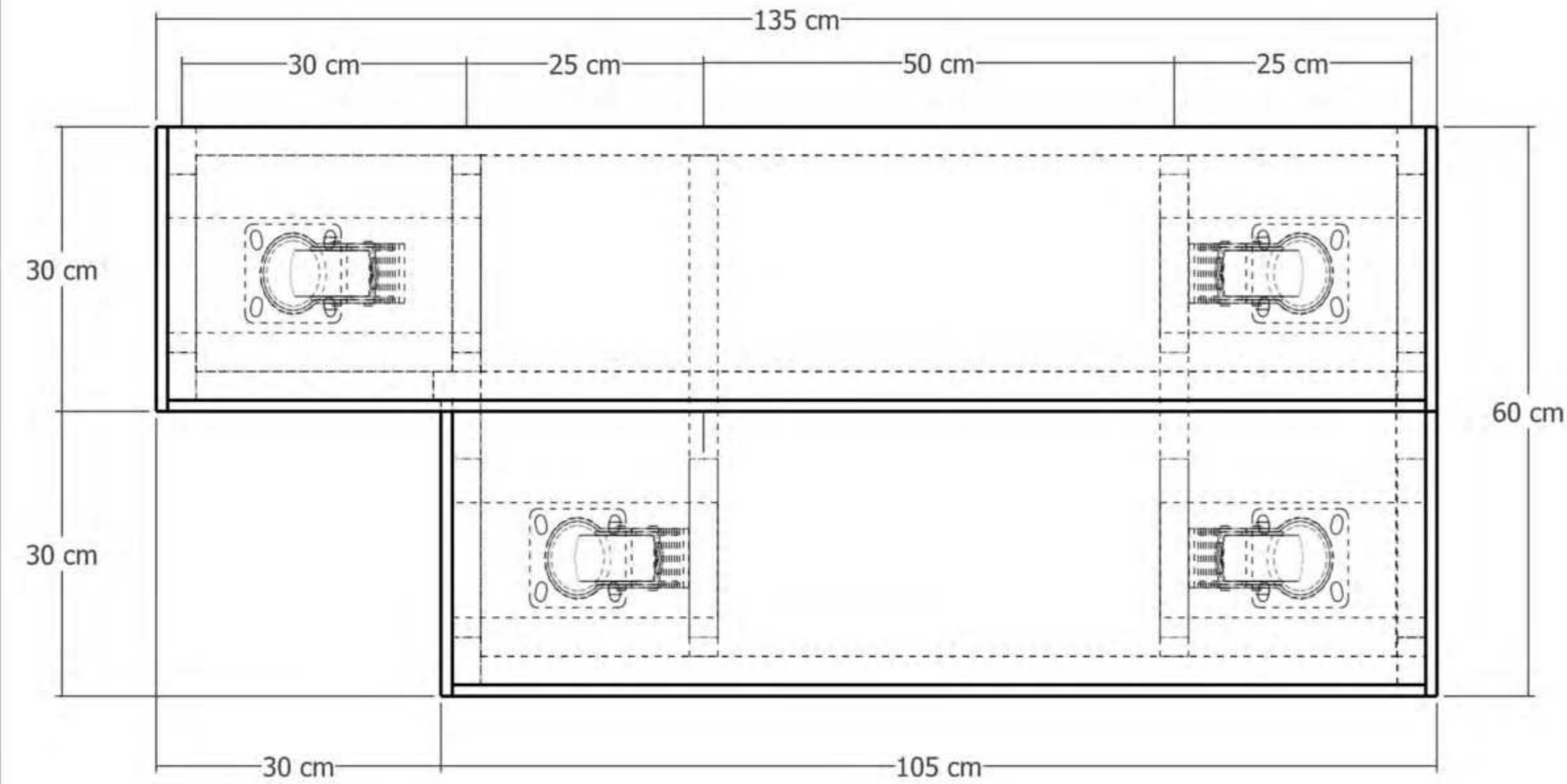
Planta
