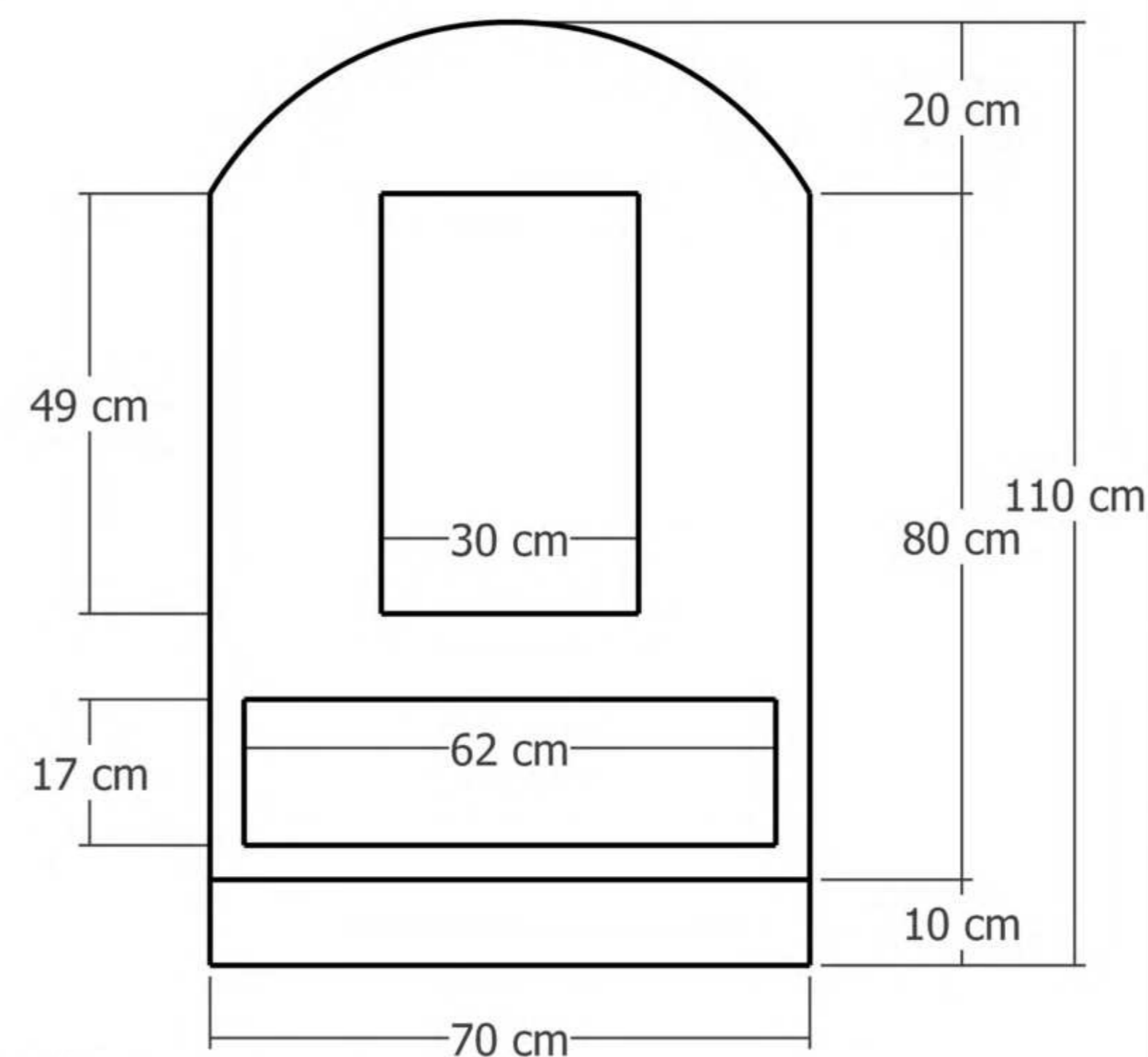
Lápide - Vista Frontal
