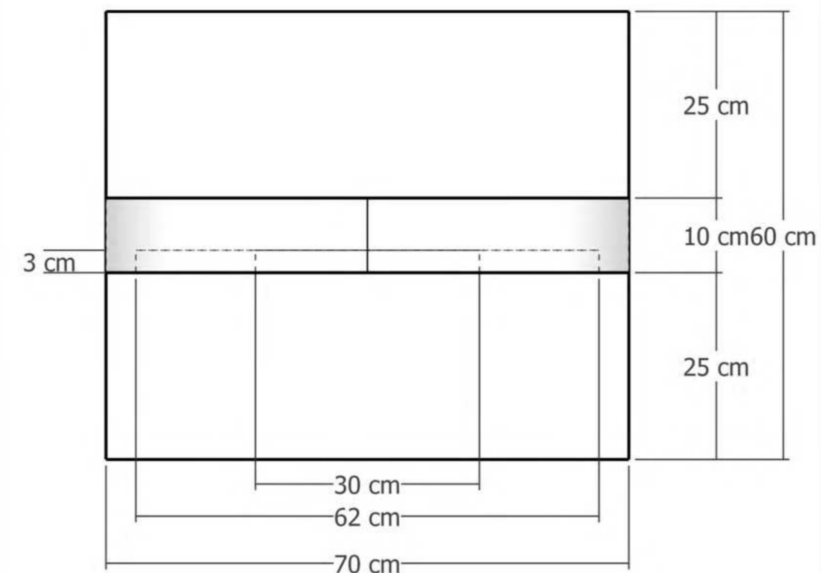
Lápide - Planta
