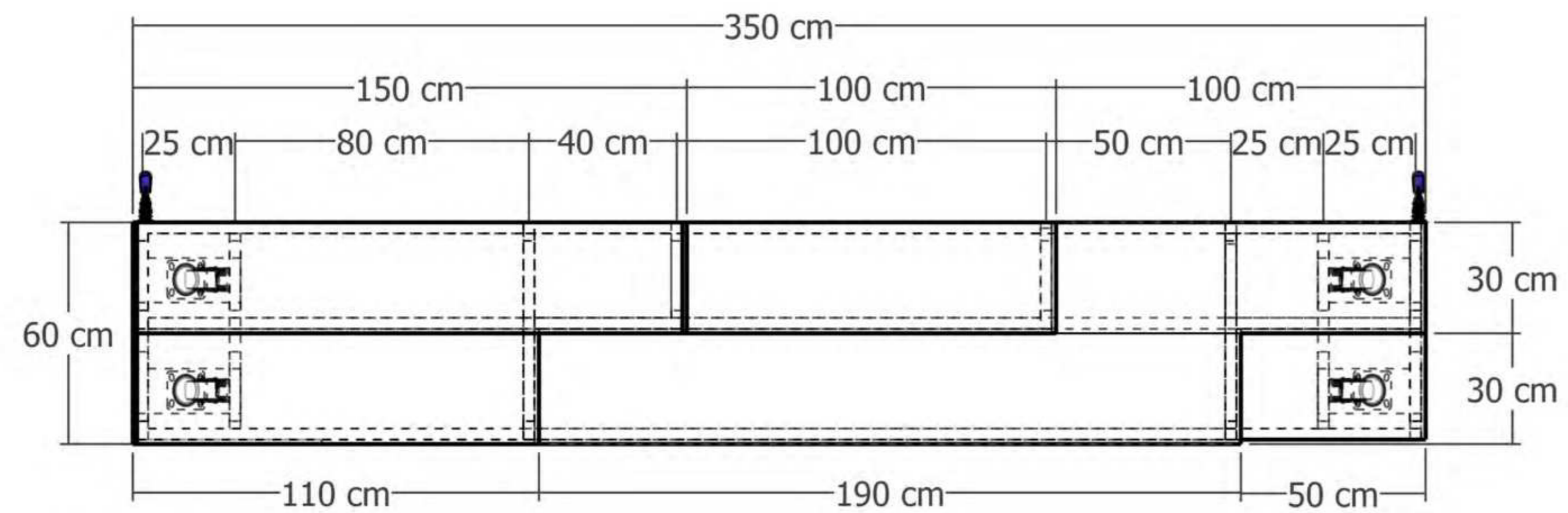
Peça B - Planta
